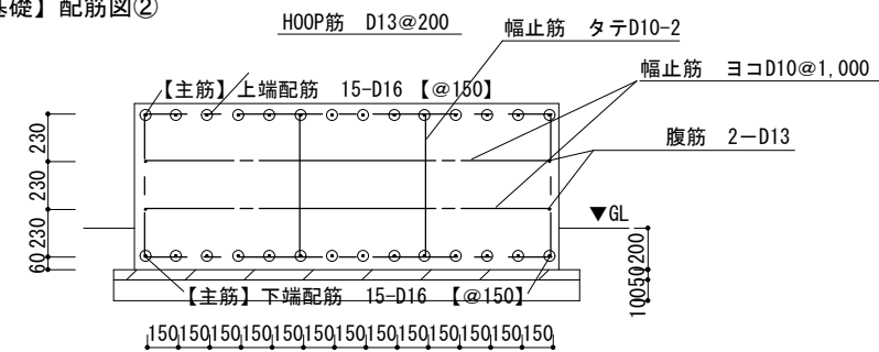
【基礎】配筋図②
