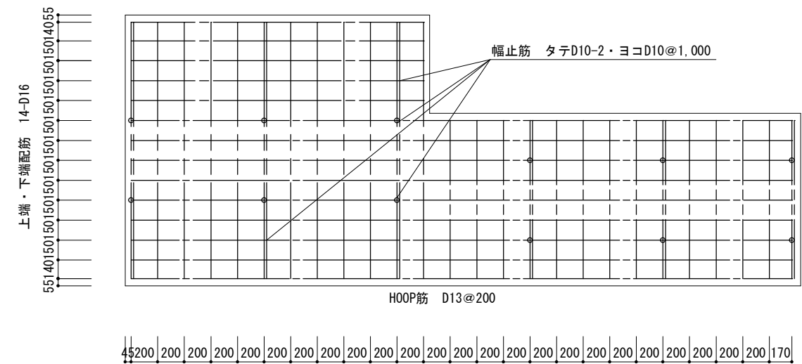
【基礎】配筋図②
