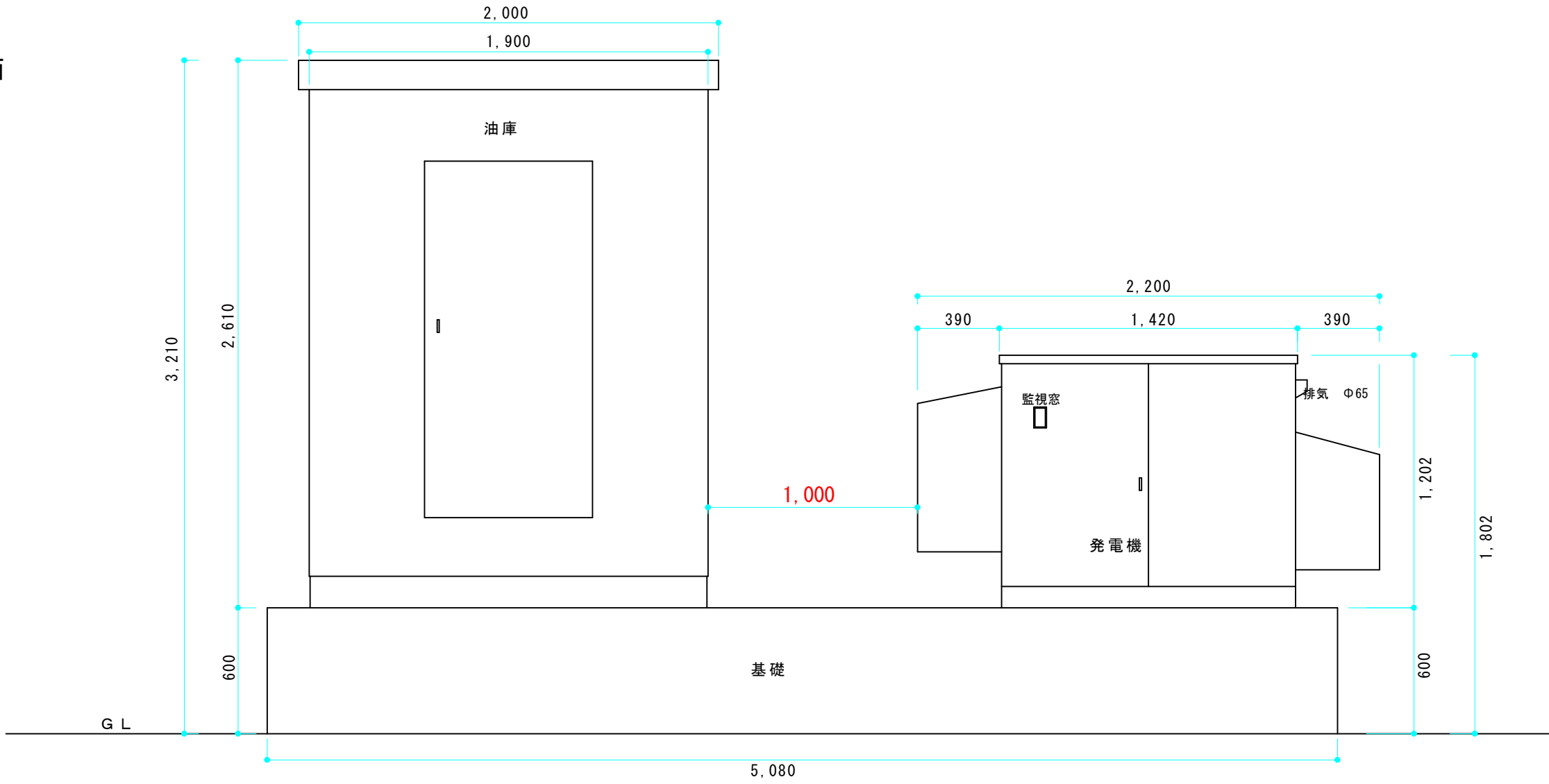
立面
